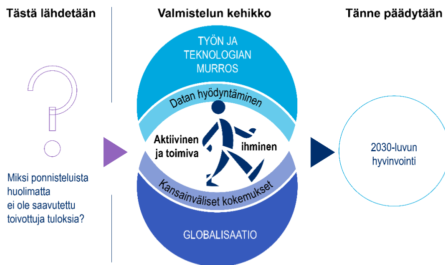
Kuva 1. Toimi-hankkeen viitekehys
